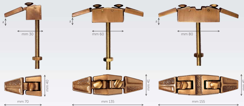
ART. 30970 - a = cm 1-2 ART. 30972 - a = cm 2-3 Perno da Ø 10 MA x 100 compreso nel prezzo
